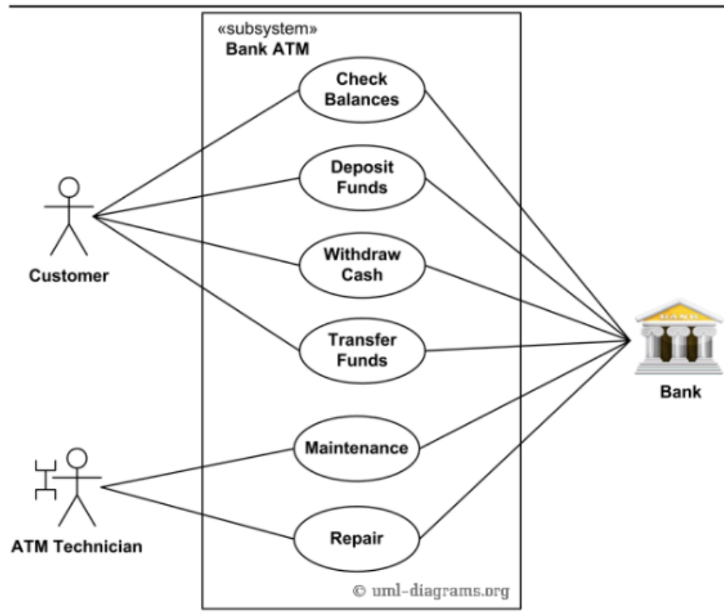
Gambar 1.3. Use-case diagram.
