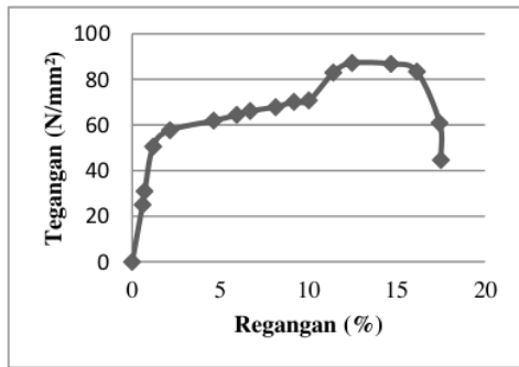
Gambar 3. Grafik tegangan dan regangan spesimen dengan induction hardening
