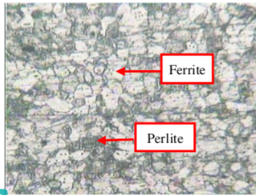
4 Gambar 6. Struktur mikro baja ST 60 dengan perlakuan flame hardening
