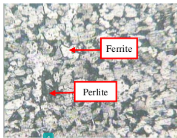
Gambar 5. Struktur mikro baja ST 60 dengan perlakuan induction hardening
