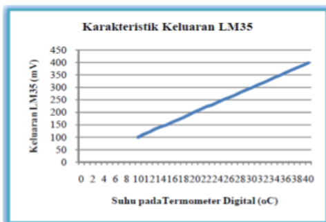
Gambar 1. Karakteristik LM 35[6]
