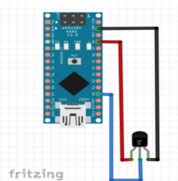
Gambar 6. Skema sensor LM 35 ke Arduino
