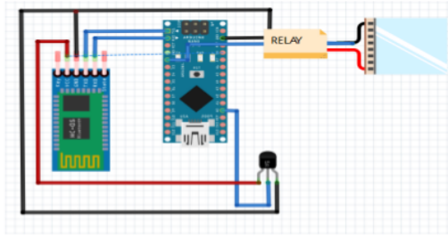
Gambar 5. Skema rangkaian
