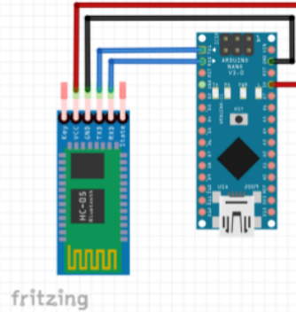
Gambar 7. Skema HC-05 ke Arduino
