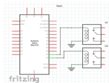
Gambar 8. Skema Relay ke Arduino
