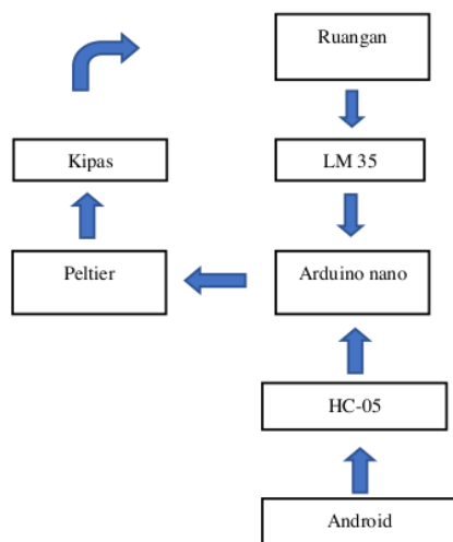
Gambar 3. Blok Diagram Sistem
