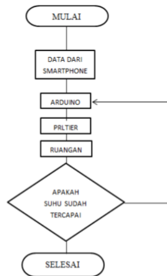
Gambar 4. Flowchart Aplikasi
