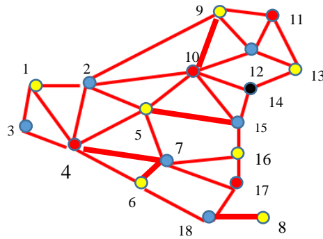
Gambar 5. Pewarnaan Simpul Graf pada wilayah Titik Distribusi
