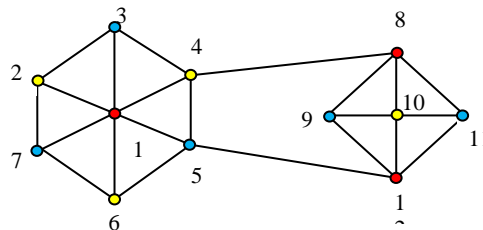
Gambar 2. Pewarnaan Simpul Menggunakan Algoritma Welch-Powell
