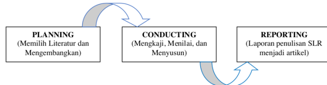
Gambar 1. Tahapan Penelitian
