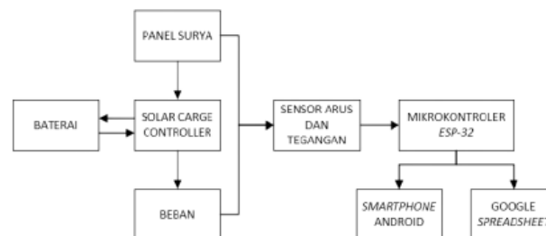
Gambar 6. Diagram blok.
