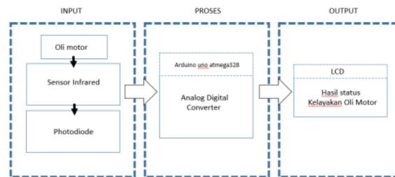
Gambar 11.1 Sistem kerja alat
