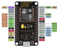
Gambar 1. NodeMCU ESP8266
