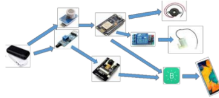
Gambar 11. Perakitan Komponen
