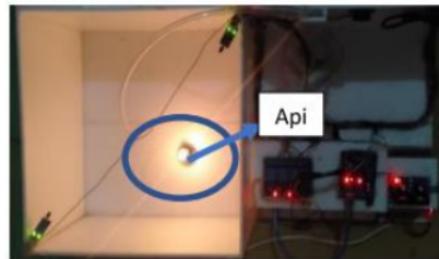
Gambar 13. Pengujian Alat
