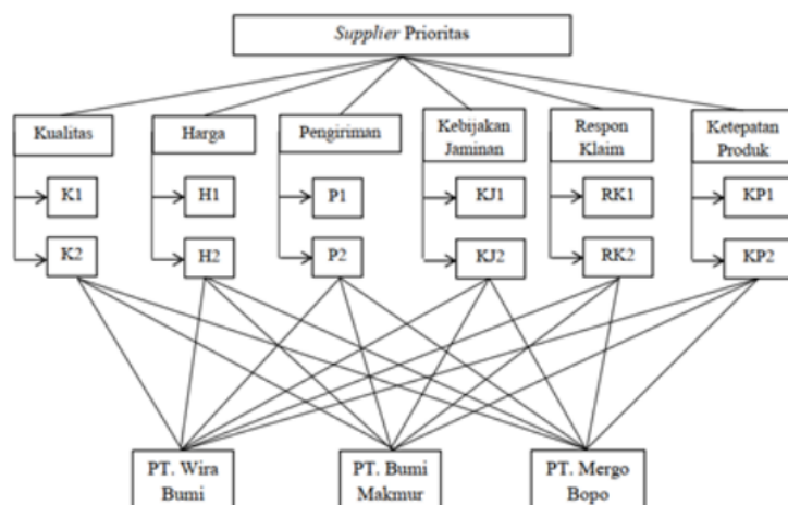
Figure 2. Struktur Hierarki
