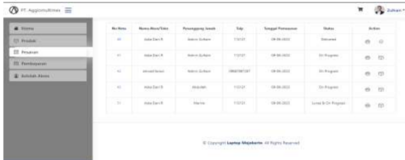
Gambar 19 Data Pesanan
