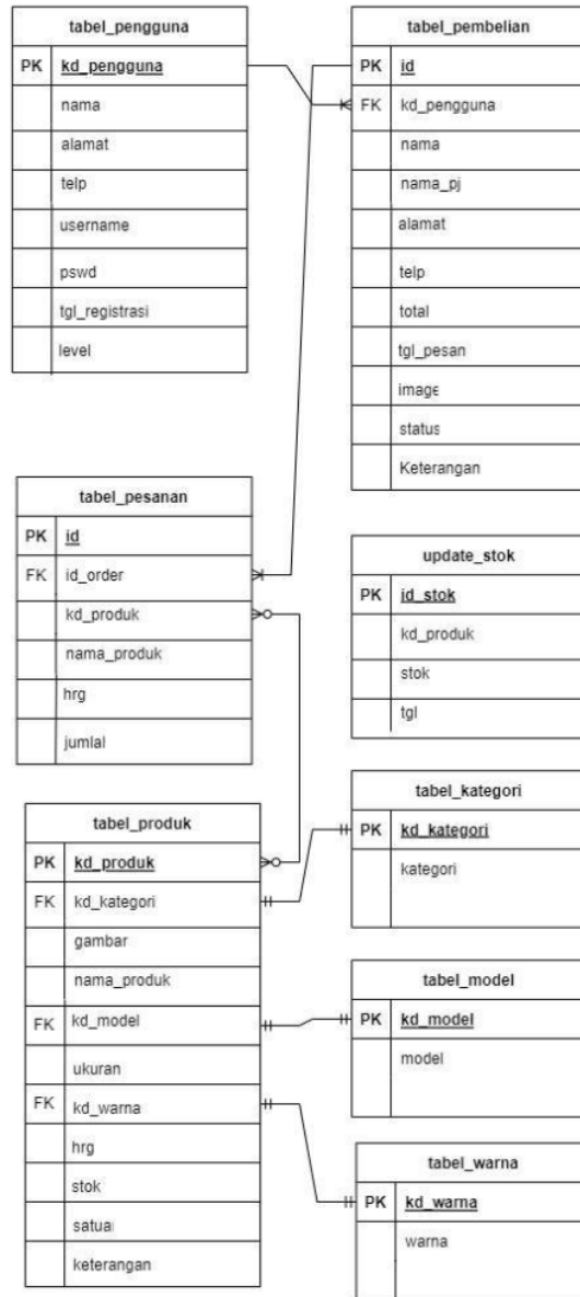
Gambar 7. Desain database
