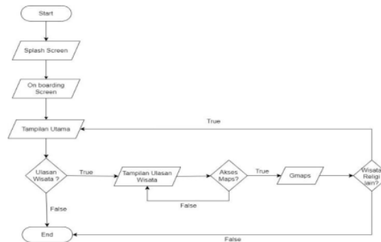
Gambar 2. Flowchart Aplikasi
