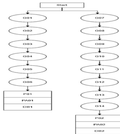
Gambar 7. Pohon keputusan
