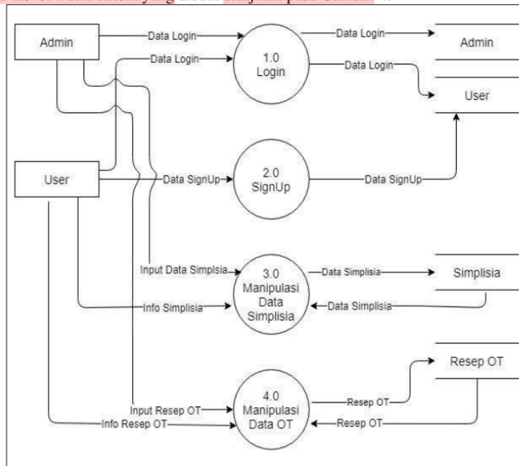
Gambar 4 DFD Level 1
