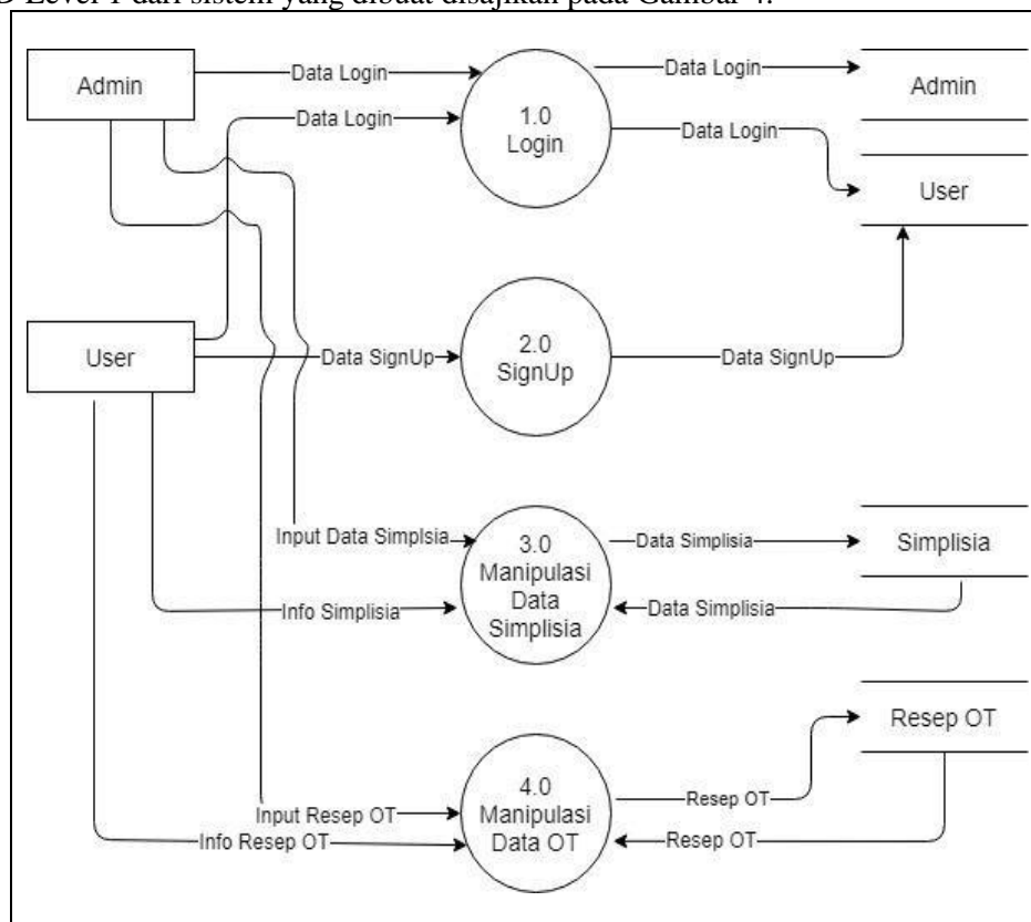
Gambar 4 DFD Level 1
