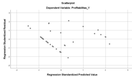
Gambar 1 Uji Heterokedastisitas
