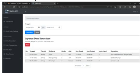
Gambar 13. Halaman Laporan
