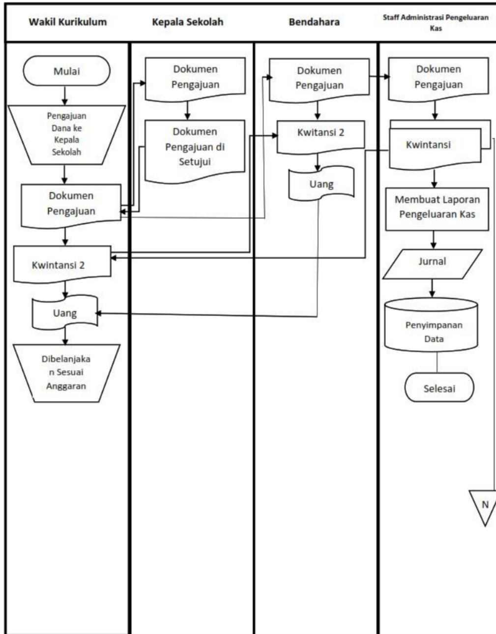
Figure 4. Flowchat Sistem Informasi Akuntansi Pengeluaran Kas Secara Tunai
