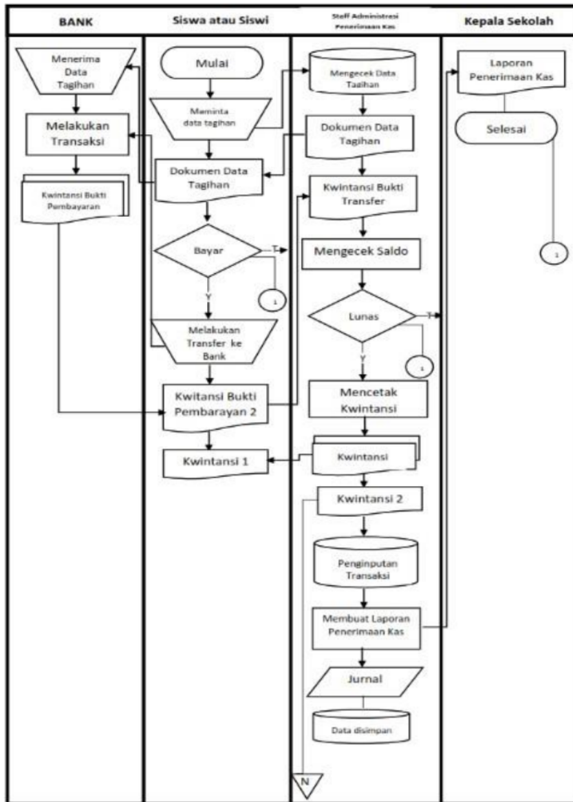
Figure 2. Flowchat Sistem Informasi Akuntansi Penerimaan Kas Secara Transfer Bersumber Dari Pembayaran Siswa atau Siswi
