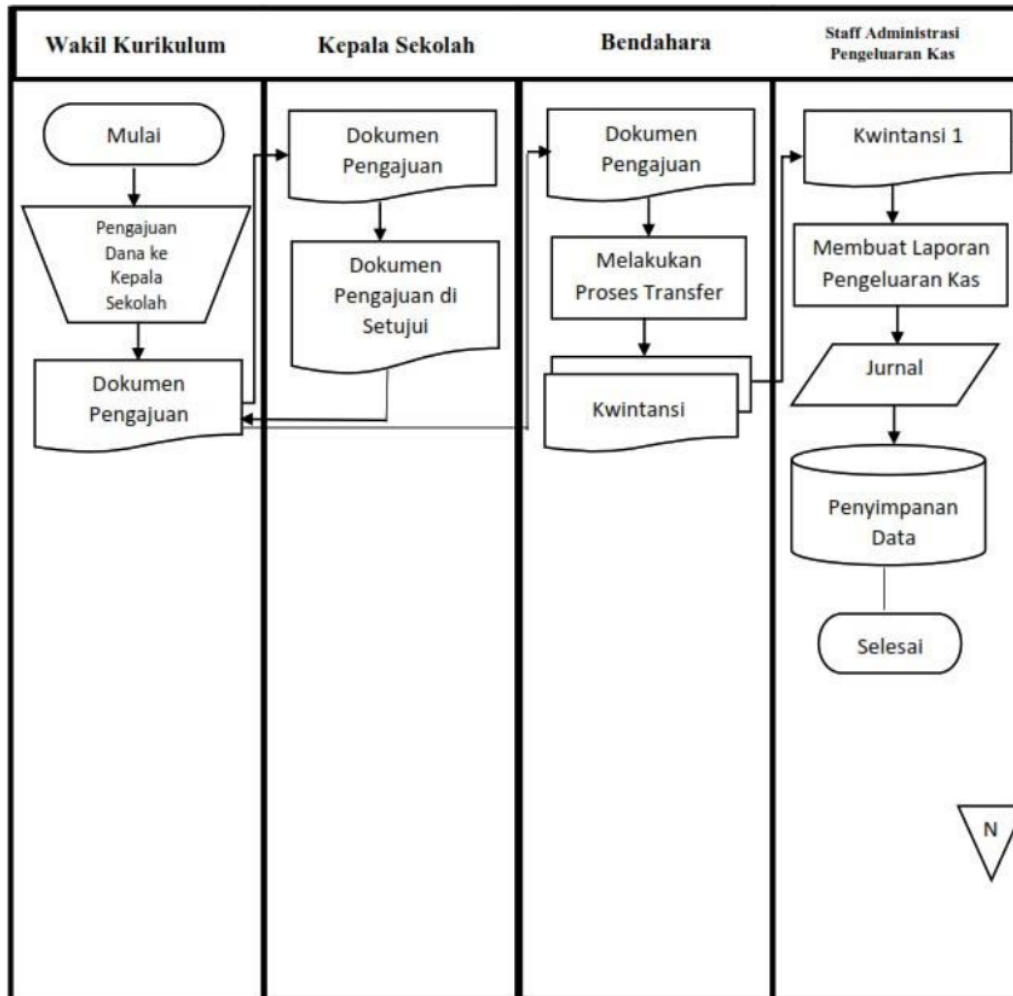
Figure 5. Flowchat Sistem Informasi Akuntansi Pengeluaran Kas Secara Transfer
