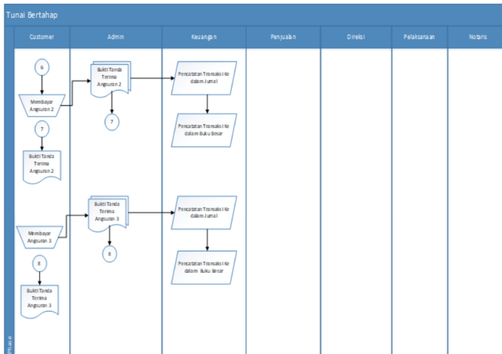
Figure 6. Flowchart Penjualan tunai dengan Pembayaran Tunai Bertahap (Lanjutan)
