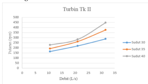
Gambar 5. Kecepatan putar turbin tk. II dengan variasi sudut pengarah
