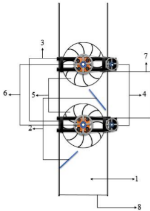
Gambar 3. Instalasi Turbin Air Bertingkat Dua
