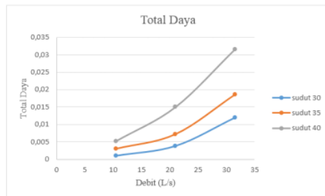
Gambar 7. Daya turbin total dengan variasi sudut pengarah
