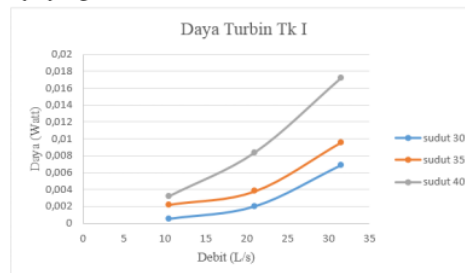
Gambar 6. Daya turbin tk. I dengan variasi sudut pengarah
