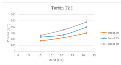
Gambar 4. Kecepatan putar turbin tk. I dengan variasi sudut pengarah
