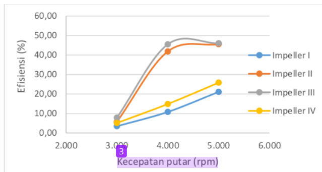
Gambar 5. Pengaruh kecepatan putar terhadap efisiensi pada variasi bentuk impeller.
