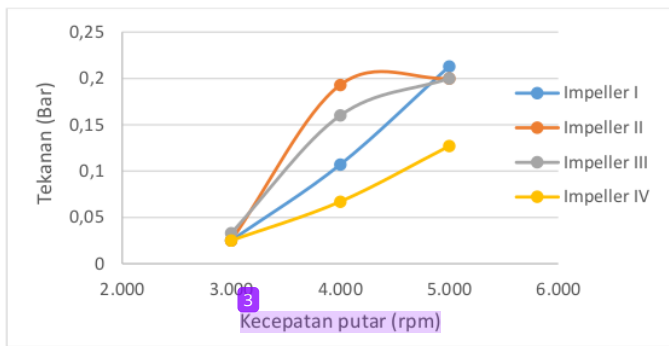
Gambar 2. Pengaruh kecepatan putar terhadap tekanan dengan variasi bentuk impeller.
