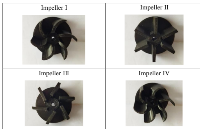
Gambar 1. Desain impeller yang diuji.
