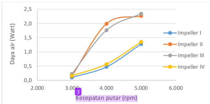
Gambar 4. Pengaruh kecepatan putar terhadap daya air pada variasi bentuk impeller
