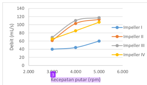
Gambar 3. Pengaruh kecepatan putar terhadap debit pada variasi bentuk impeller.
