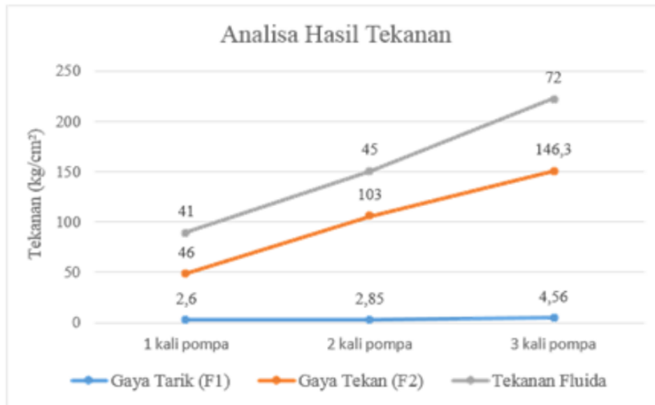
Figure 5. Grafik Hasil uji tekanan pada tracker hidrolik
