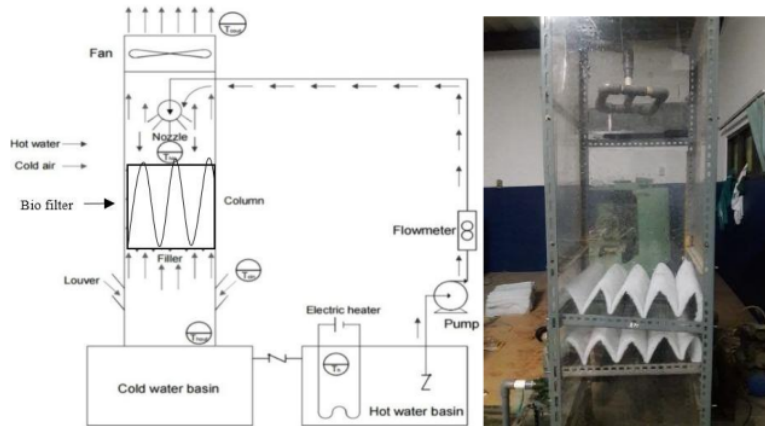
Gambar 1. Instalasi Pengujian [10]
