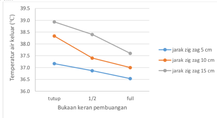
Gambar 4. Grafik temperatur air keluar rata – rata
