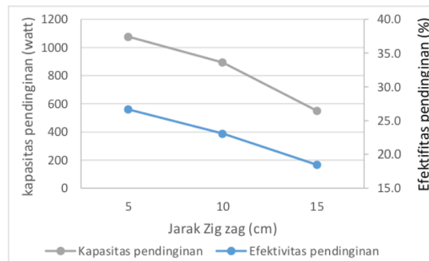
Gambar 8. Grafik perbedaan kapasitas pendinginan dan efektifitas pendinginan
