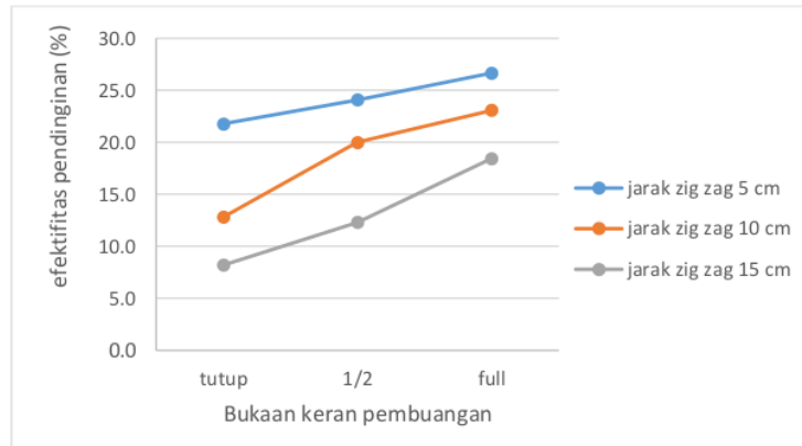
Gambar 7. Grafik efektifitas pendinginan
