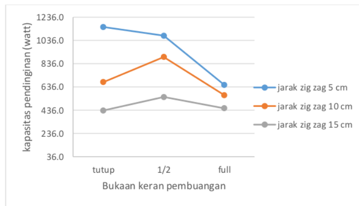
Gambar 6. Grafik kapasitas pendingin
