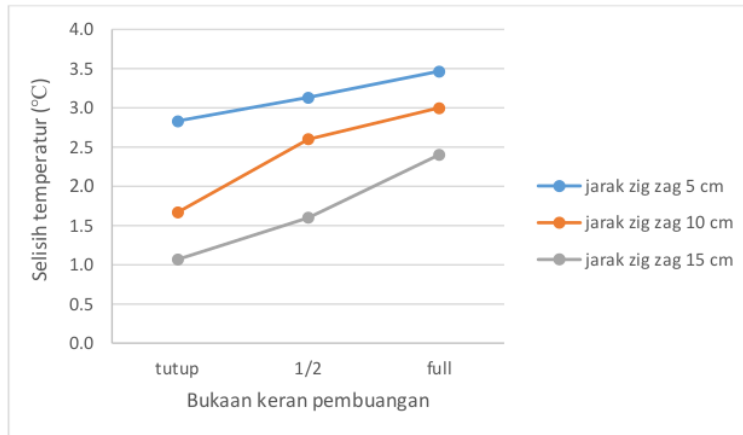
Gambar 5. Grafik selisih temperatur
