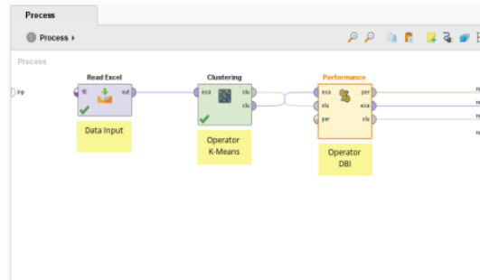
Gambar 1. Desain Lembar Kerja Clustering Rapidminer
