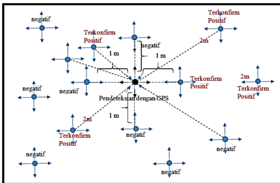
Gambar 2. Model Penyebaran Pasien Terkonfirmasi Covid 19 Melalui Penggambaran Graf
