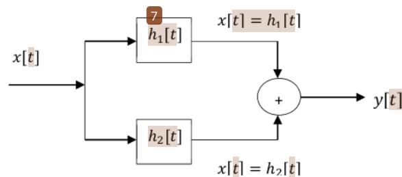
Gambar 4 Receiver terhubung secara paralel [6]
