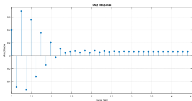
Gambar 10 Step Respon sinyal SET dengan n = 1
