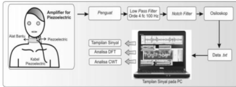
Gambar 3. Diagram blok subsistem perancangan perekaman Carotid Pulse .
