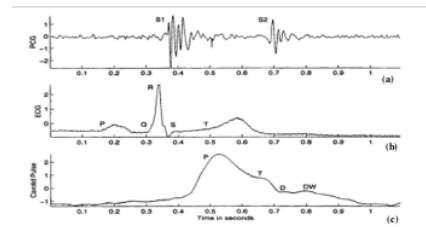
Gambar 1 Perekaman secara simultan sinyal PCG (a), ECG (b), dan Carotid Pulse (c) (Ranagayyan,2002)
