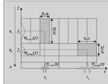
Gambar.2. Resolusi waktu dan frekuensi CWT [5]
