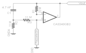
Gambar 4. Rangkain Amplifier Piezoelectric
