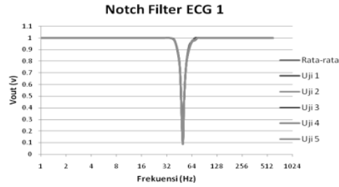
Gambar 9. Grafik Hasil Uji Notch Filter 1
