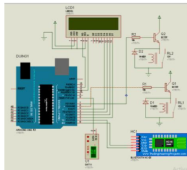
Gambar 7. Rangkaian Skematik Alat
