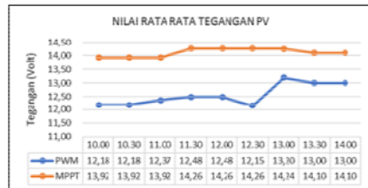
Gambar 4. Rata-Rata Tegangan PV menggunakan PWM dan MPPT (Beban>200W)
