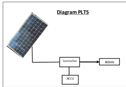
Gambar 2. Blok Diagram PLTS
