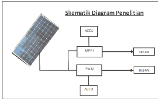
Gambar 3. Skematik Pelaksanaan Penelitian
