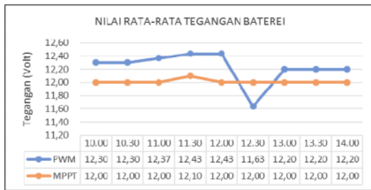
Gambar 5. Rata-Rata Tegangan Baterai menggunakan PWM dan MPPT (Beban>200W)
