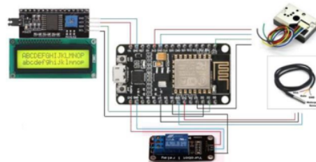
Gambar 1. Wiring Komponen
