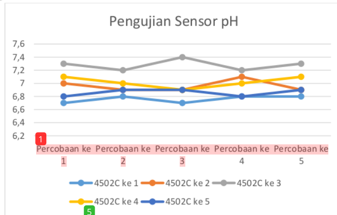
Gambar 8. Grafik Pengujian Sensor pH
