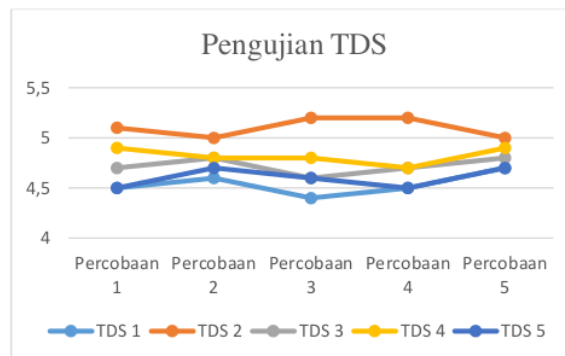
Gambar 7. Grafik Pengujian Sensor TDS
