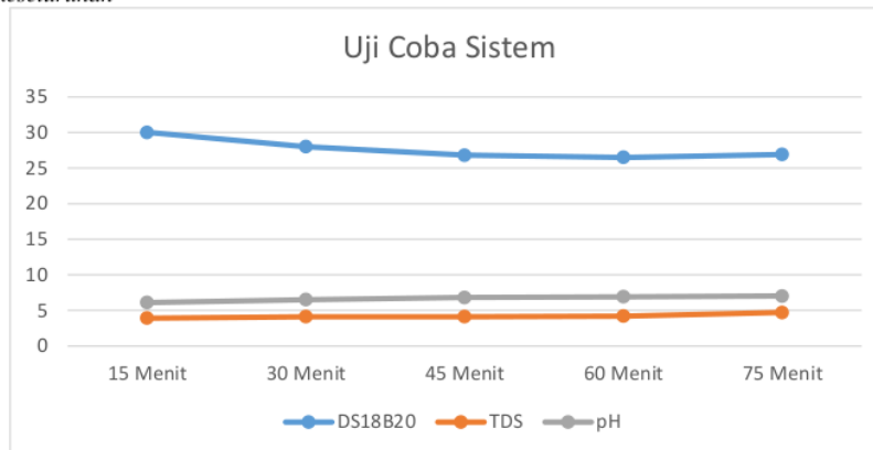
Gambar 9. Grafik Pengujian Sistem
