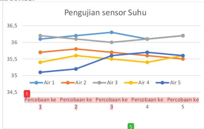
Gambar 6. Grafik pengujian sensor suhu
