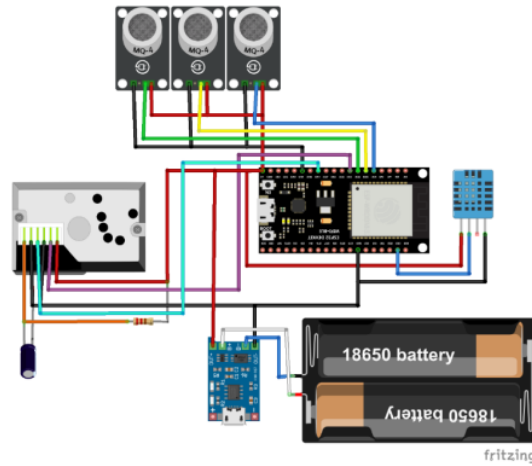
Gambar 2. Perancangan hardware dengan software Fritzing
