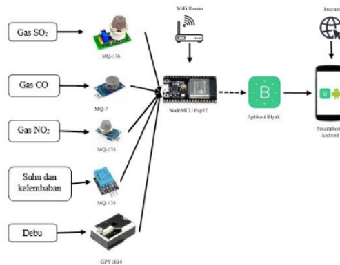
Gambar 4. Blok diagram alat yang dibuat
