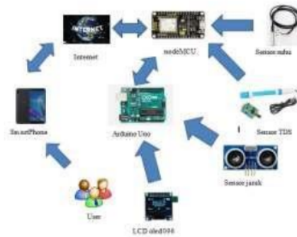
Gambar 2. Diagram blok sistem
