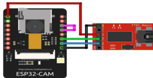
Gambar 6. Rangkaian Kamera ESP32 dengan USB to serial (FTDI)
