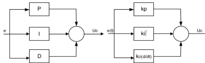
Gambar 3. Struktur Kontroler PID.
